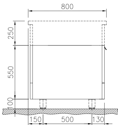
Zij aanzicht
